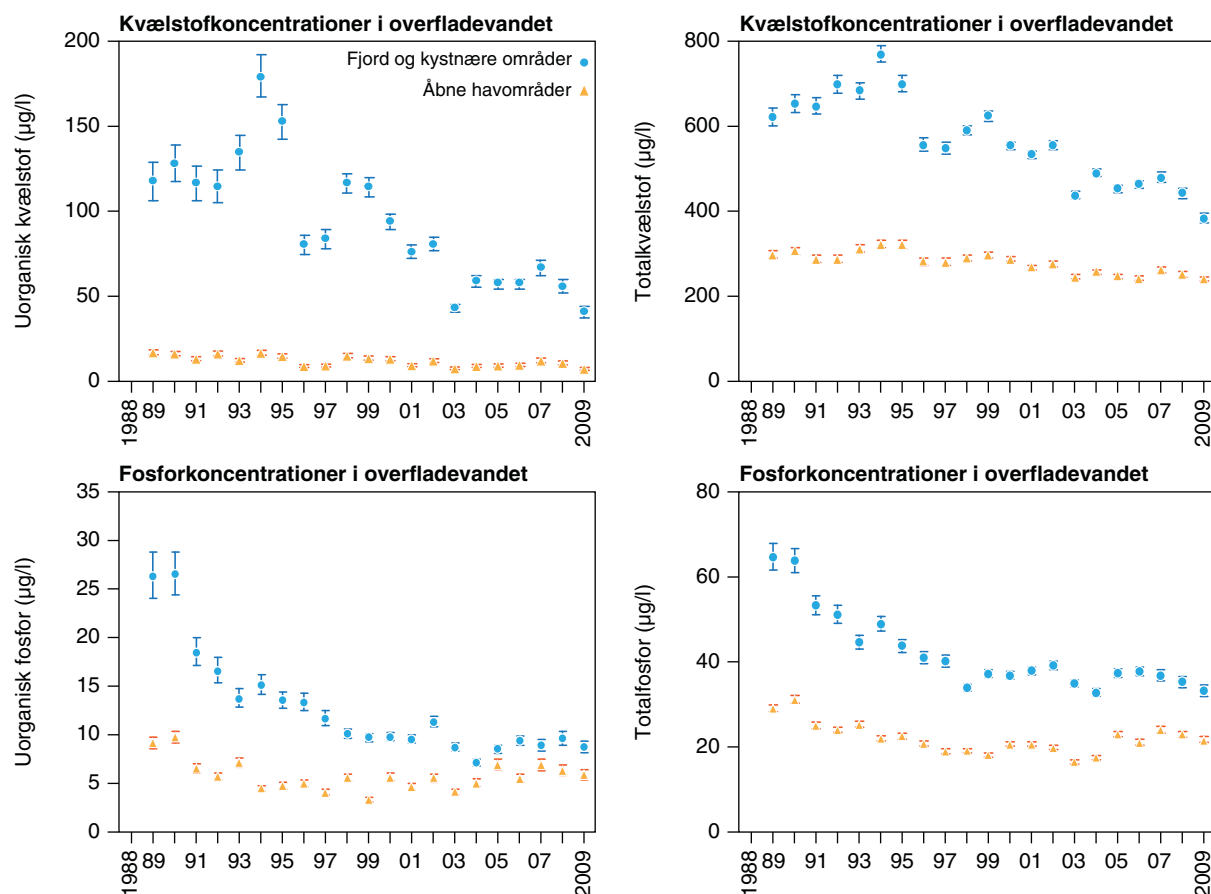
Figur 9.2. Årsmiddelkoncentrationer af uorganisk kvælstof, total kvælstof, uorganisk fosfor og total fosfor i overfladevandet. Middelkoncentrationerne er afbildet med angivelse af 95% konfidensgrænser. Fjorde og kystnære områder er i alle grafer afbildet med cirkler, mens åbne havområder er markeret med trekanter (Petersen & Hjort (red) 2010).
