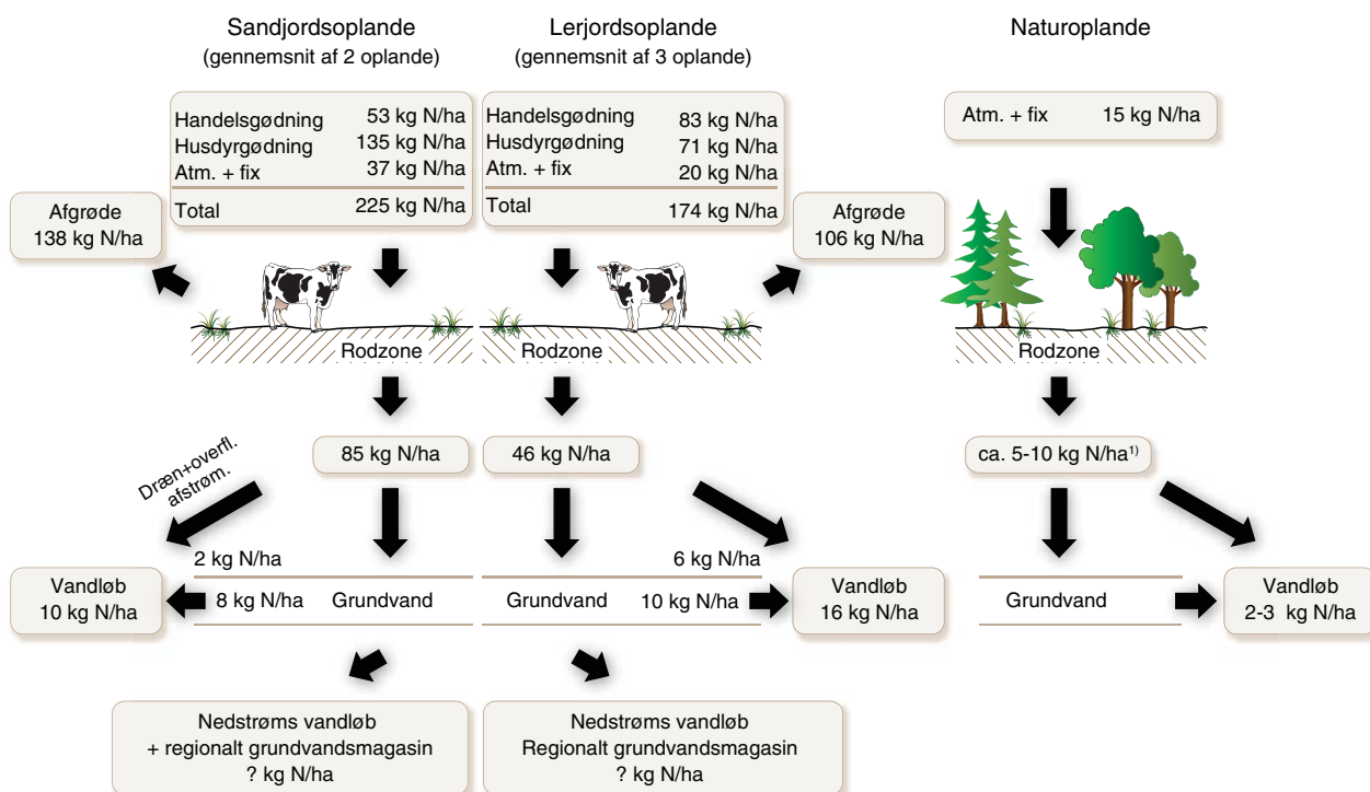
Figur 2.13. Skematisering af kvælstofkredsløbet i henholdsvis dyrkede lerjords- og sandjordsoplande samt naturoplande for de hydrologiske år 2003/04-2008/9 (og tilhørende landbrugspraksis 2004-2008). Tilførsel og fraførsel af kvælstof er baseret på data fra interviewundersøgelsen og udvaskningen er modelberegnet med N-LES4 for alle marker i oplandet. NB! Vandløbs-transport i landbrugsoplandene er korrigeret for naturarealer og spildevandsudledning, dvs. transporten repræsenterer det dyrkede areal incl. spredt bebyggelse (Grant et al. 2010). 1) Intervallet for naturarealer, 5-10 kg N/ha henviser til udvaskningen fra hhv. gammel skov og landbrugsjord omlagt til natur, herunder skov.
