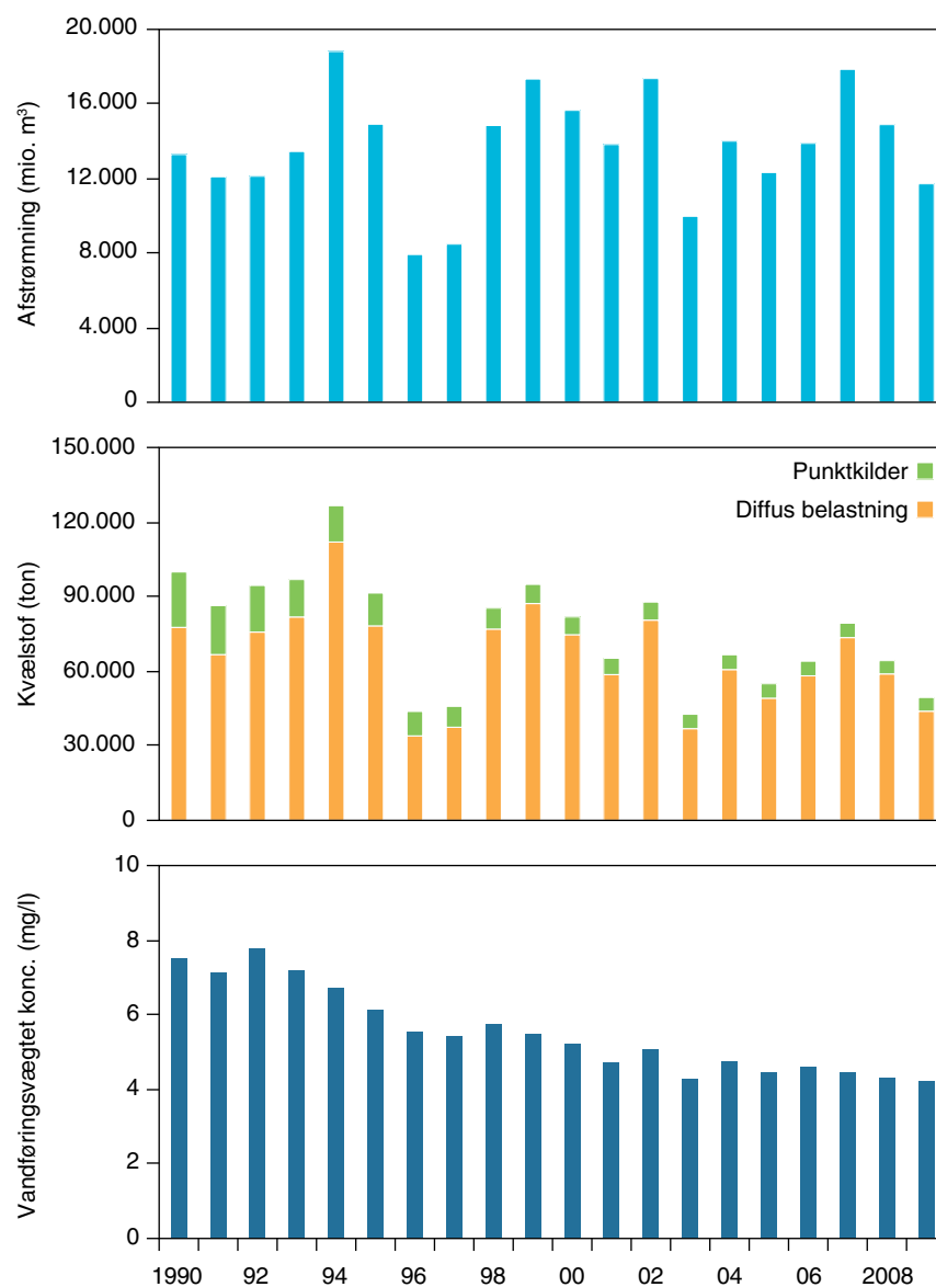
Figur 2.1. Udvikling i ferskvands-afstrømning (øverst), kvælstoftilførsel (midterst) og vandføringsvægtet kvælstofkoncentration i det afstrømmende ferskvand til havet omkring Danmark (nederst), 1990-2009. Kvælstoftilførslen er fordelt på diffuse kilder (inkl. spildevand fra spredt bebyggelse) og spildevand fra punktkilder (Wiberg-Larsen et al. 2010).
