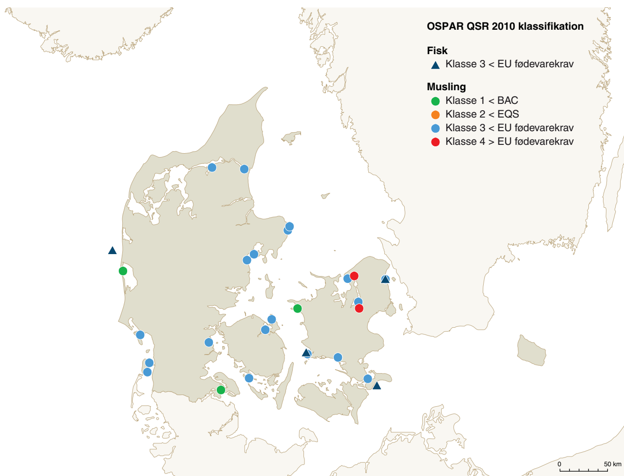
Figur 9.9. Vurdering af cadmium, bly og kviksølv i prøver af muslinger, fisk og sediment efter OSPAR's vurderingskriterier (Petersen og Hjorth (red.) 2010). BAC: Baggrundsniveau, OSPAR.
