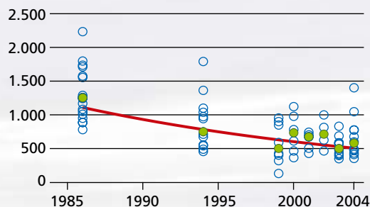
Tunup natsiisa sisamat inorlugit ukiullit orsuanni PCB-ip allanngoriartornera
