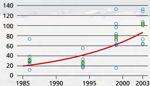
1985-2003-imi Tunup puisaasa tinguisa qalliuti-nik fluoritalinnik akuu.
