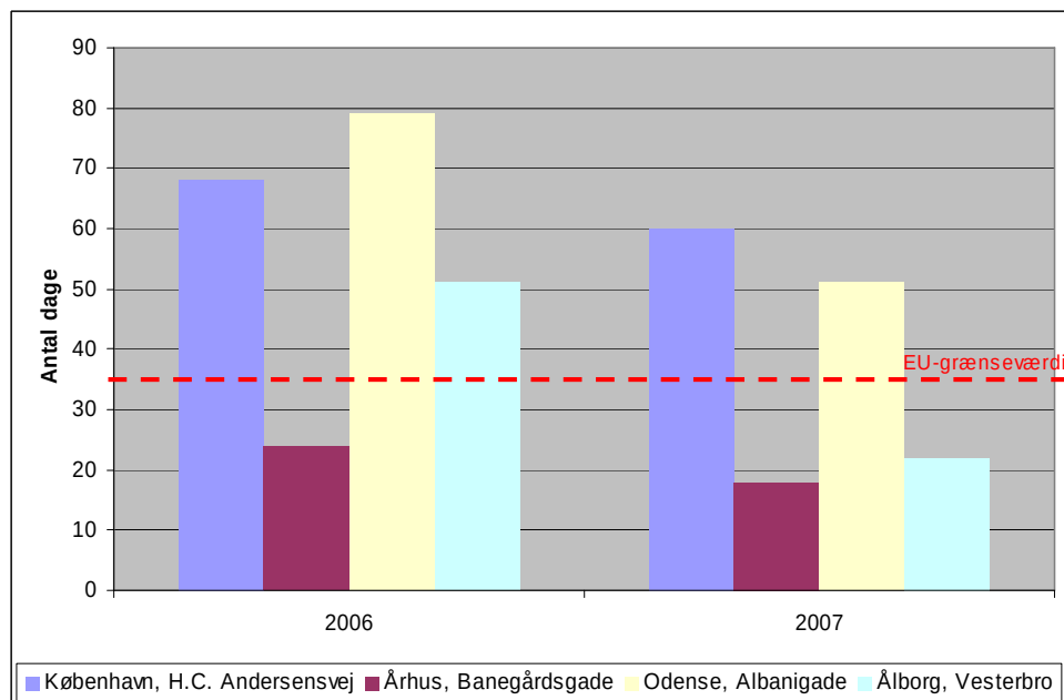
Figur 2. Antal dage om året med overskridelser af EU's grænseværdi for partikler i byluften. Grænseværdien på 50 µg/m 3 målt som døgnmiddelværdien for partikler (PM 10 ) må højst overskrides 35 dage om året.
