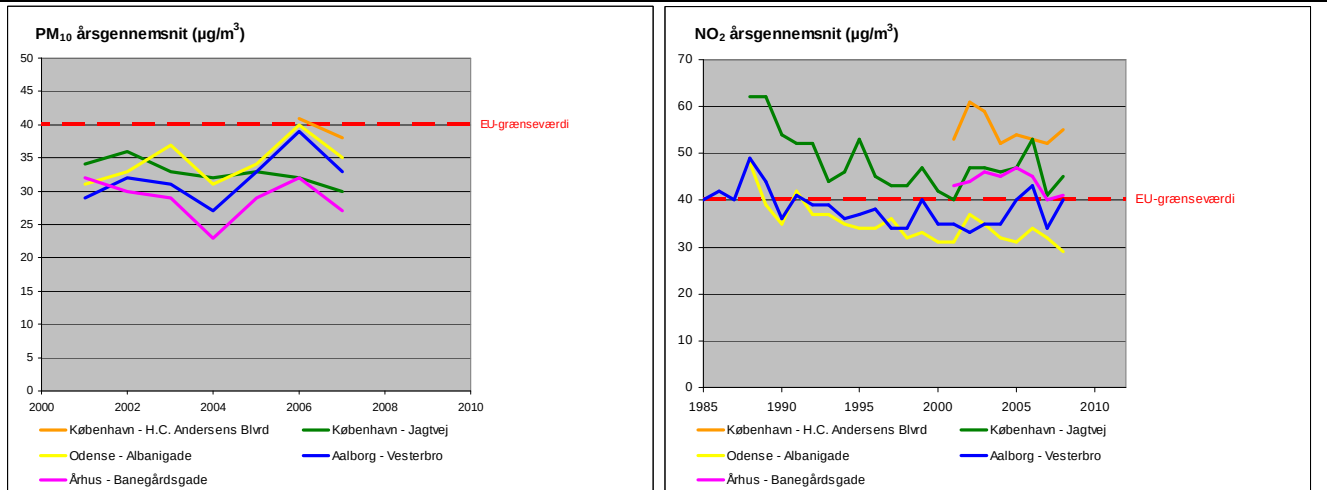
Figur 1. Luftens koncentration af partikler (PM 10 ) og nitrogen dioxide (NO 2 ) på målestationer i København, Århus, Odense og Aalborg. EU's grænseværdier er også angivet (PM 10 gælder fra 2005 og NO 2 fra 2010).
