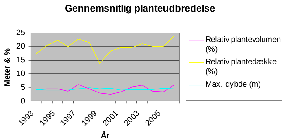
Figur 2 Undervandsvegetationens arealudbredelse, volumen samt dybdegrænse i danske søer. Kilde: Danmarks Miljøundersøgelser
