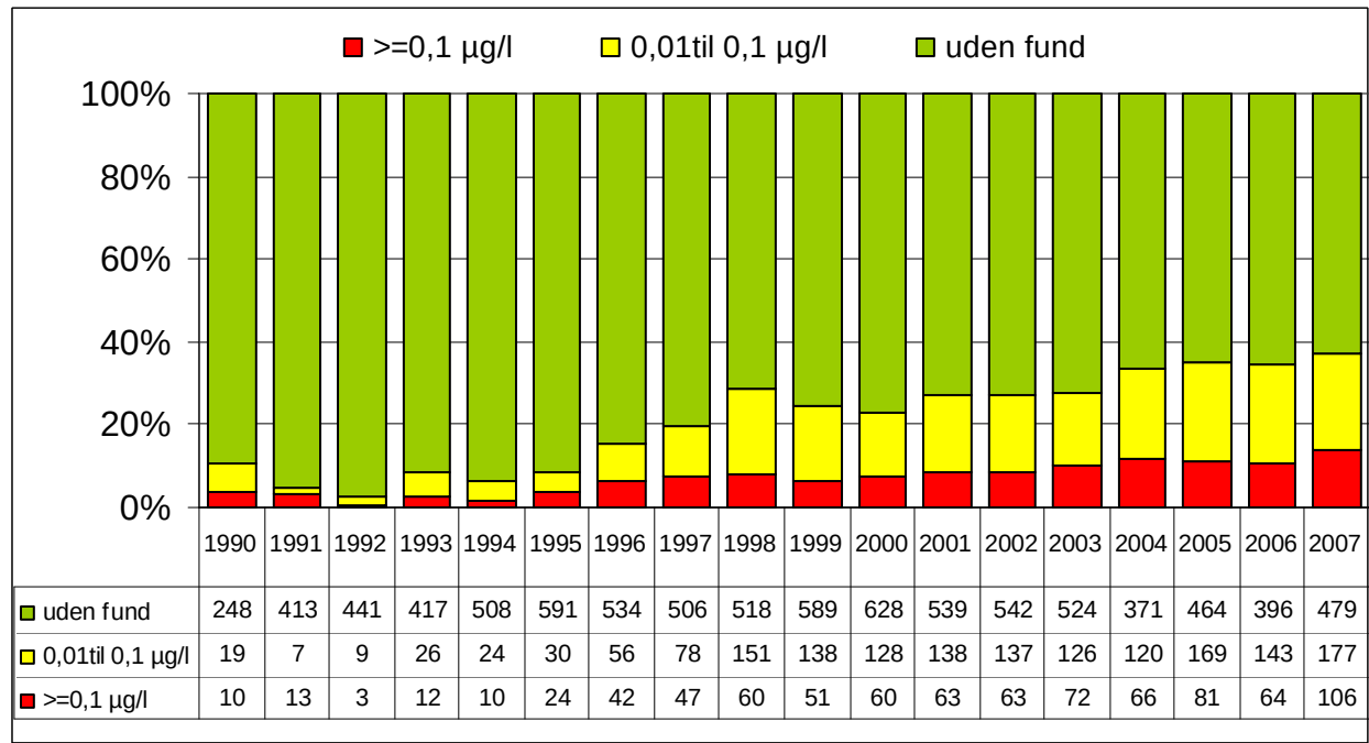
Figur 1 Fund af pesticider i grundvandet. Figuren viser antal indtag (boringer) med fund af pesticider over 0,1 µg/l, der er grænseværdien for pesticidindhold i drikkevand, antal indtag med fund i intervallet 0,01 til 0,1 µg/l og antal indtag uden fund. Kilde: De Nationale Geologiske Undersøgelser for Danmark og Grønland (GEUS)
