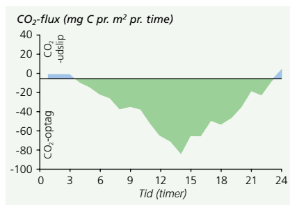
Figur 7 Kantlynghedens CO 2 -udveksling i løbet af et døgn (beregnet som gennemsnit af 5. og 6. juli 2000). I fire nattetimer er der svagt CO 2 -udslip mens resten af døgnet har netto CO 2 -optag. Bemærk at nedadrettet CO 2 -flux regnes negativt mens en opadrettet regnes positiv.
